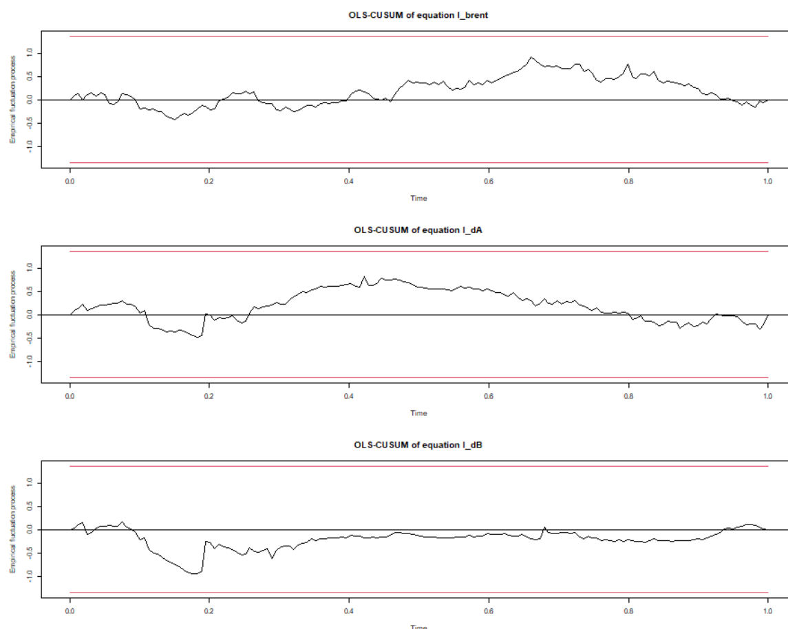
Figura 4: Gráficos OLS-CUSUM para as três equações do sistema (VAR em níveis auxiliar). As linhas vermelhas são as bandas de confiança a 5%.
